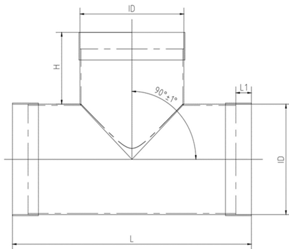
AGRU TEE
